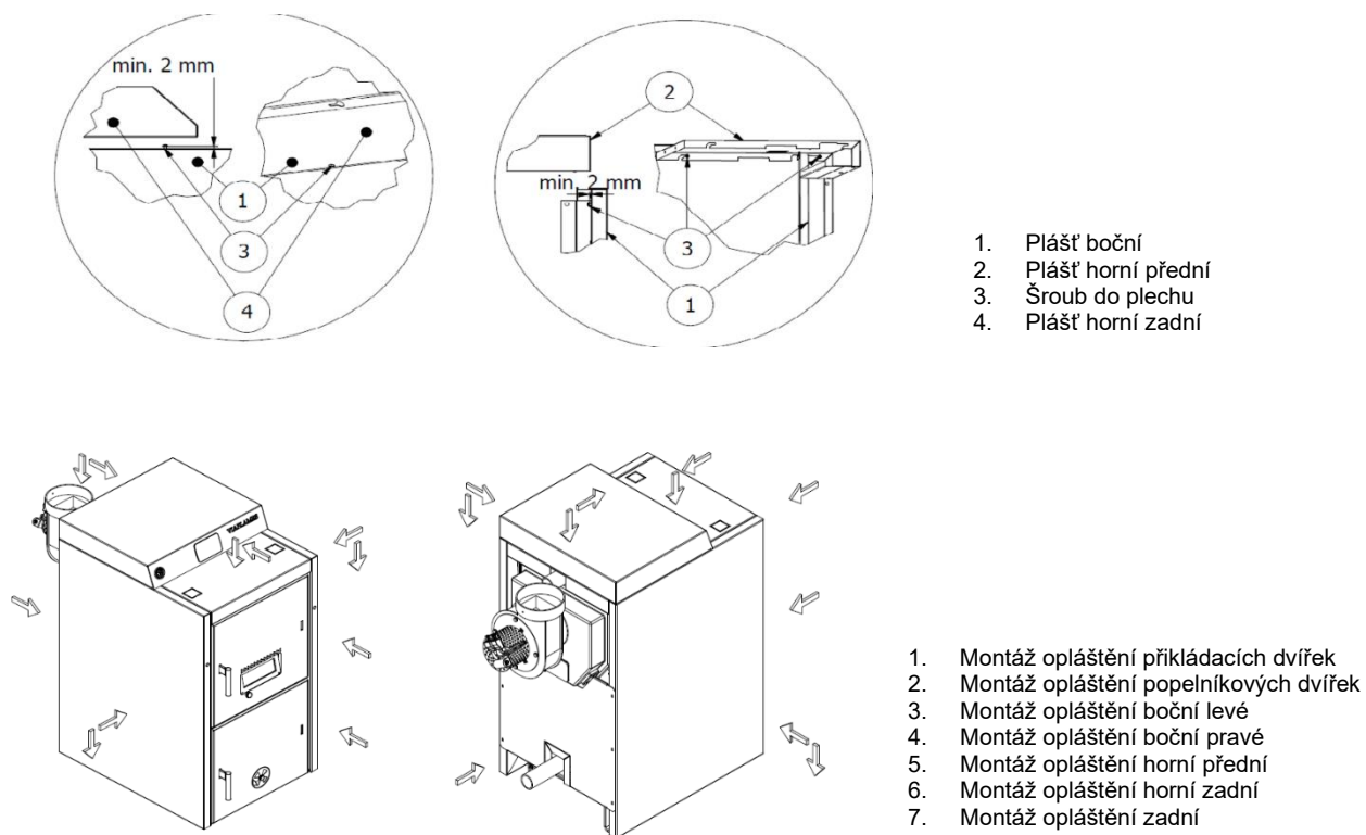
Obr.20 Postup montáže opláštění
