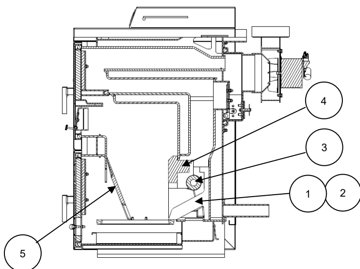
Obr. 13 Umístění žárobetonových tvarovek a šikmého roštu ve spalovací komoře kotle E22 ECO
