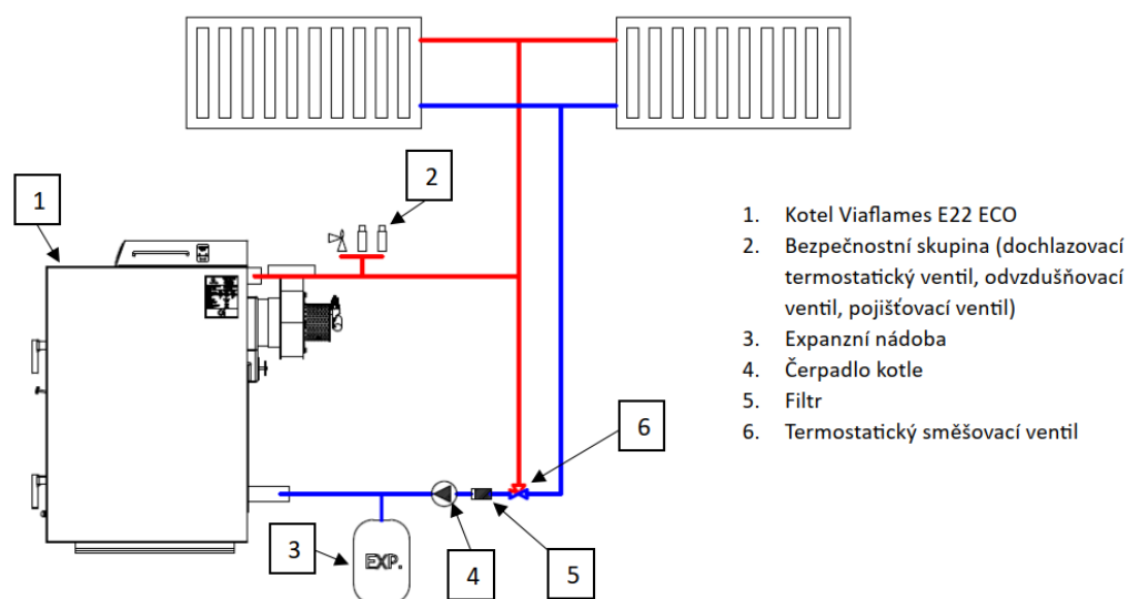
Schéma nuceného zapojení s termostatickým směšovací ventilem a havarijním dochlazováním
