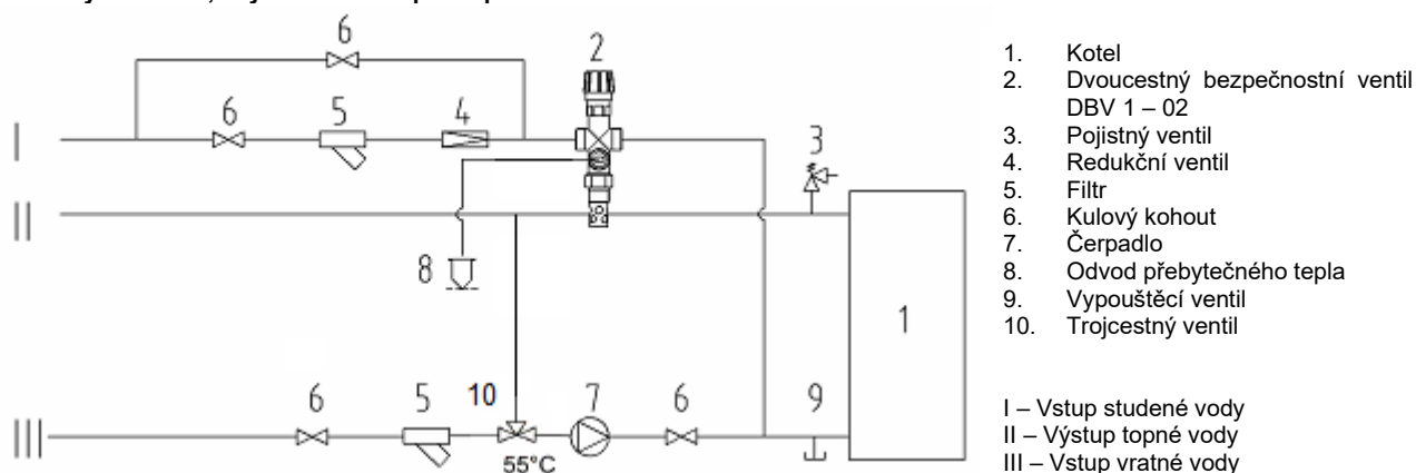
Obr. 7 Doporučené schéma zapojení dvoucestného bezpečnostního ventilu DBV 1 - 02
