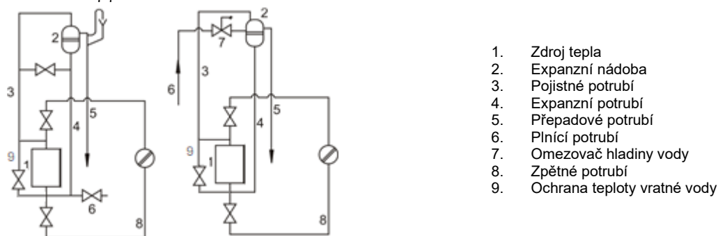
Obr. 8 Příklad zapojení otevřené expanzní nádoby
